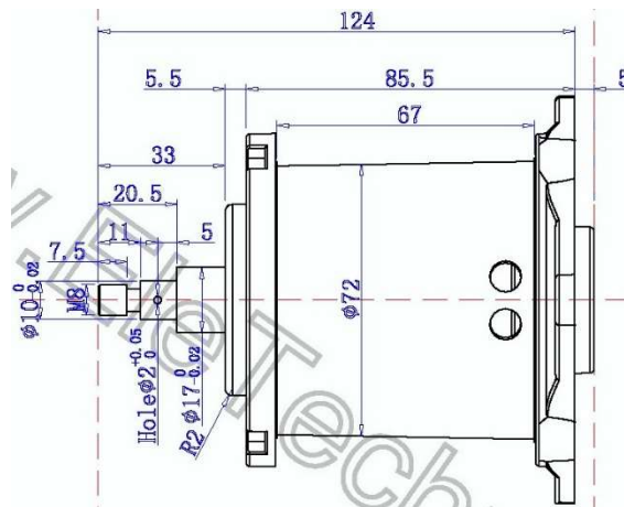
台阶轴
